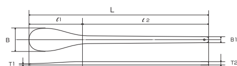
ハイテクスパテラ・ハイテクスパテラハード 寸法表
